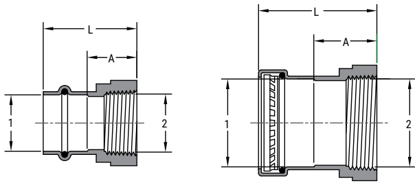
SP608 CU P X FT ADPT CPLG
