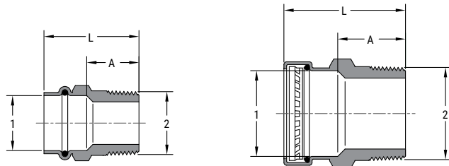
SP607 P X MT ADPT CPLG
