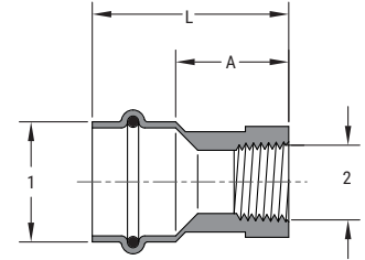
SP608R CU P X FT RED ADPT CPLG
