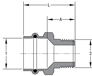
SP607R P X MT RED ADPT CPLG
