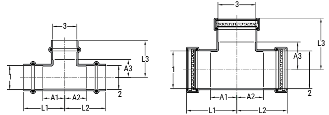
SP690 CU P x P x P Tee
