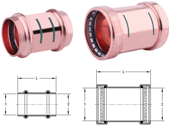
SP605 CU P X P NO STOP CPLG
