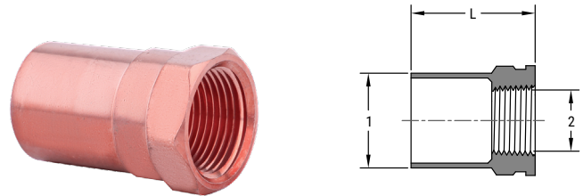
SP603R MS x FT ADPT CPLG
