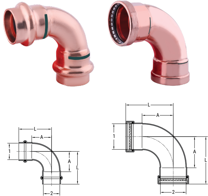
SP690 CU P X P 90 ELL
